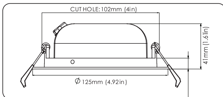
Airtight Gimbal
